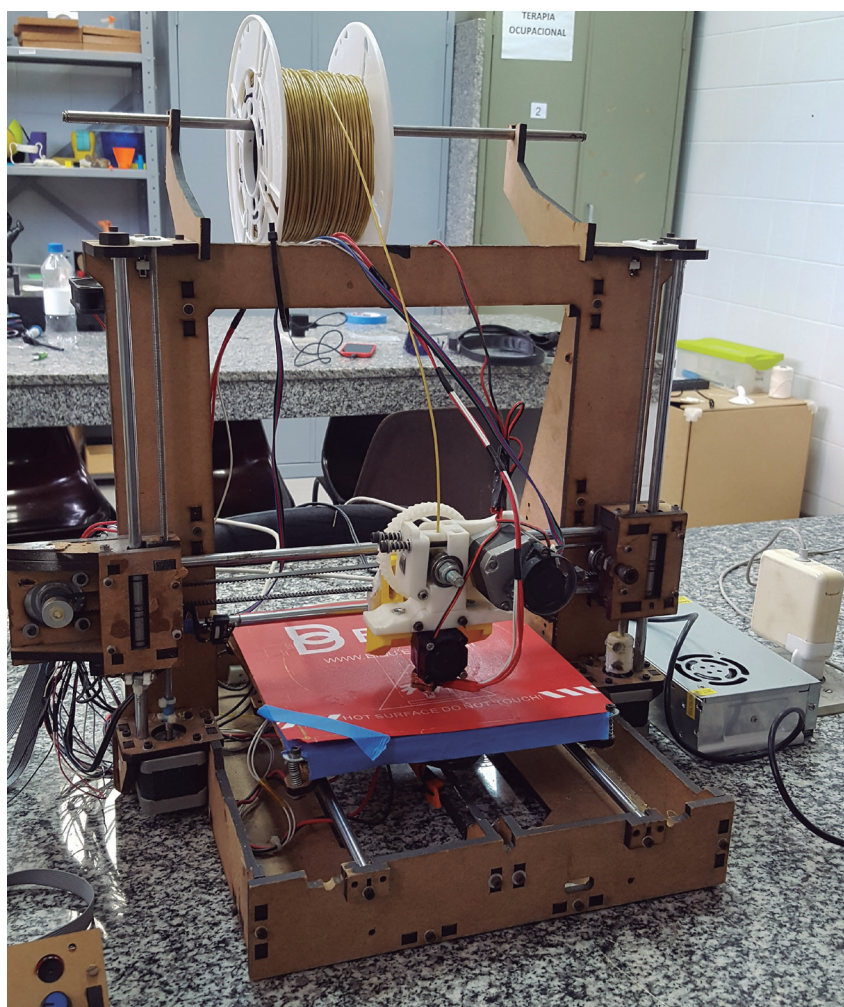
A impressora 3D utilizada pelos pesquisadores da UFES para imprimir órteses e próteses.
