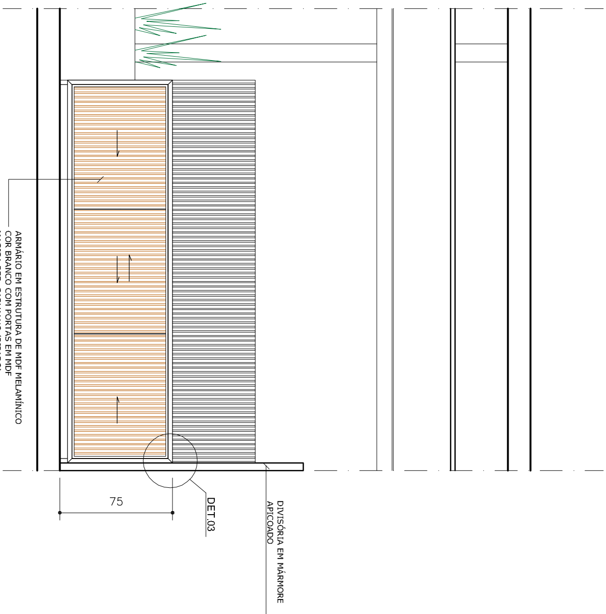
VISTA 'CC' - ATENDIMENTO (ARMÁRIO EXTERNO)
