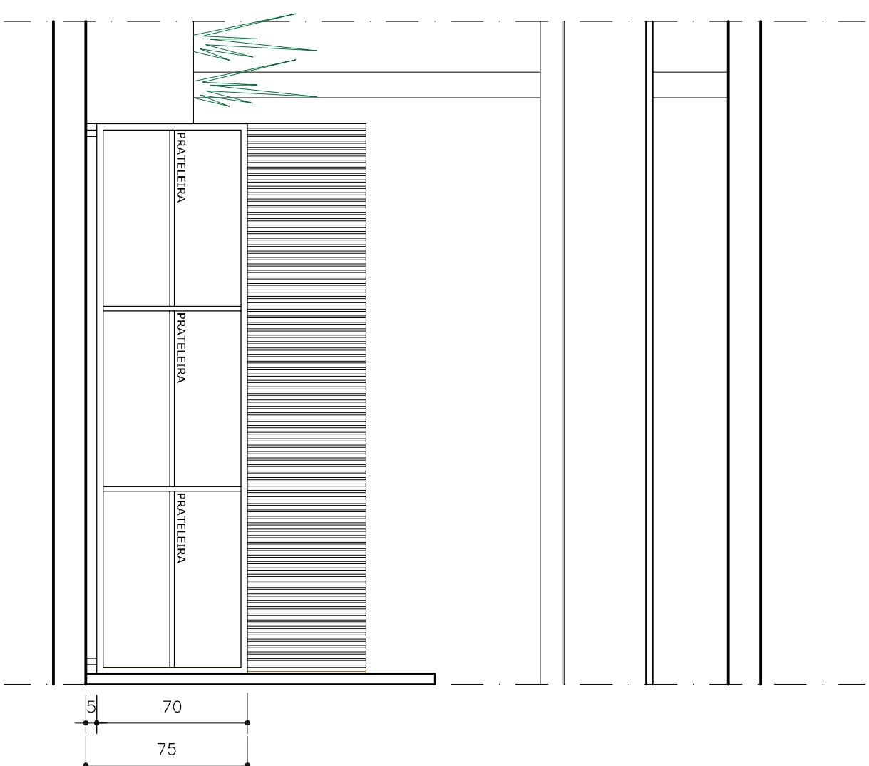
VISTA 'CC' - ATENDIMENTO (ARMÁRIO INTERNO)
