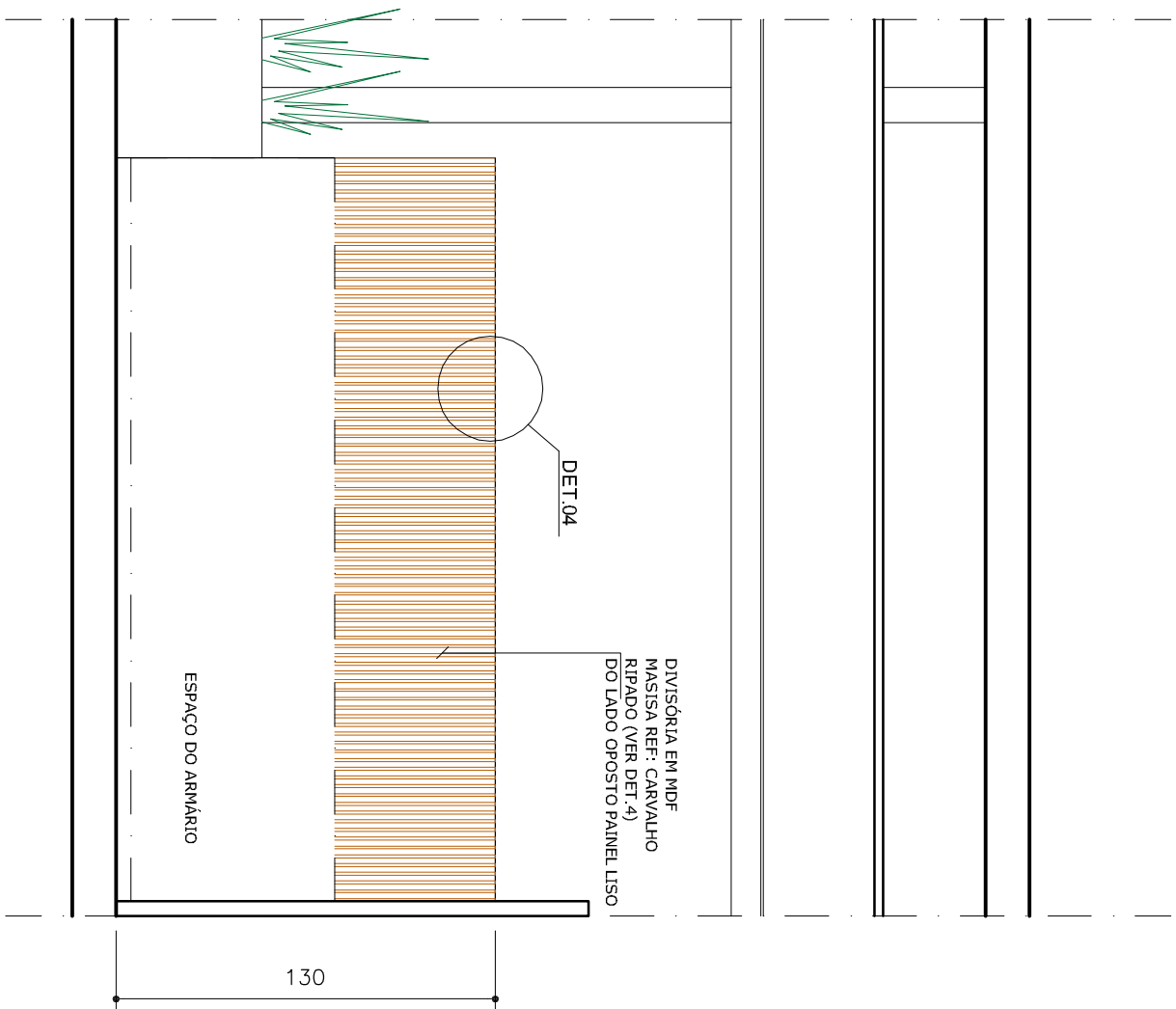
VISTA 'CC' - ATENDIMENTO (DIVISÓRIA)
