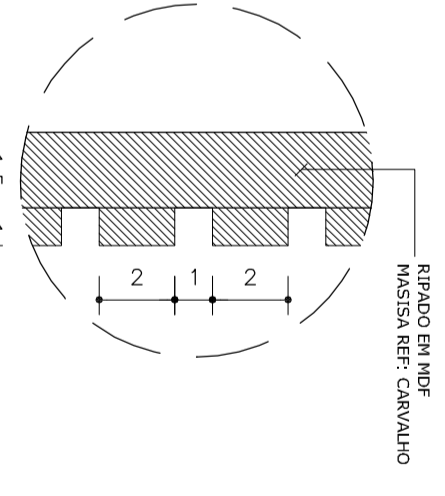
DETALHE 1 - RIPADO ESC.: 1/2
